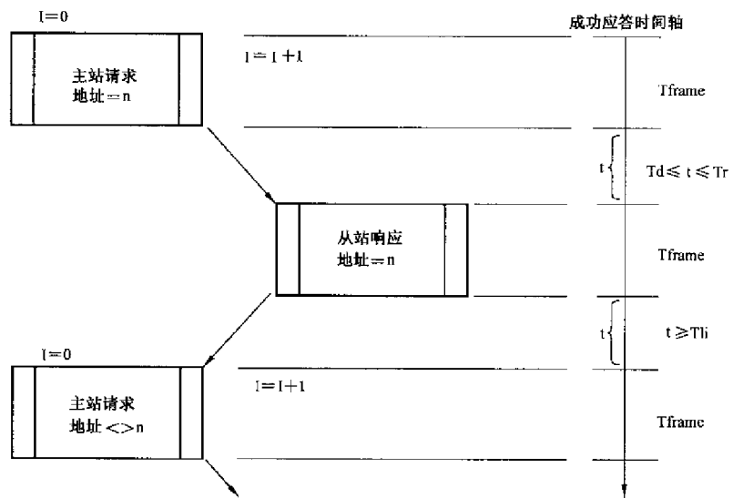
图 4 主站请求成功时序图
