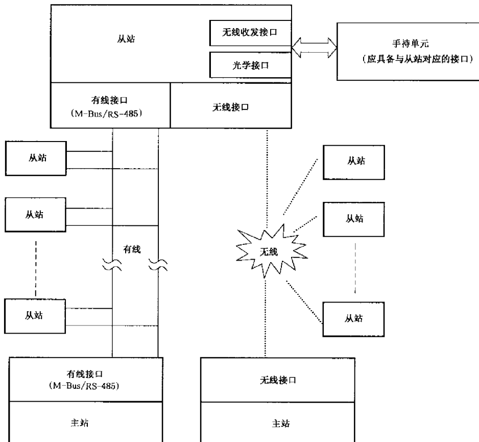
图 1 集抄系统示意图
