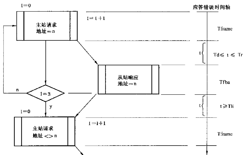
图 6 主站请求应答错误失败时序图
