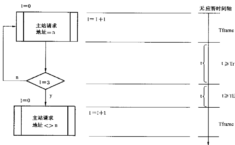
图 5 主站请求无应答失败时序图
