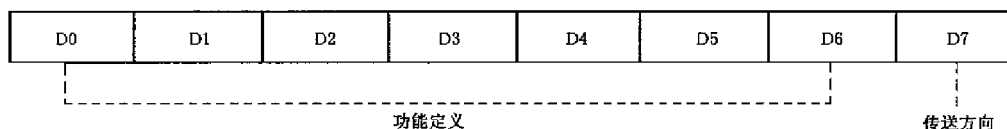
图 3 控制码格式
